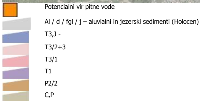
Slika 8: Geološka zgradba Dravelske doline (Vir: GeoZS, 2017).
