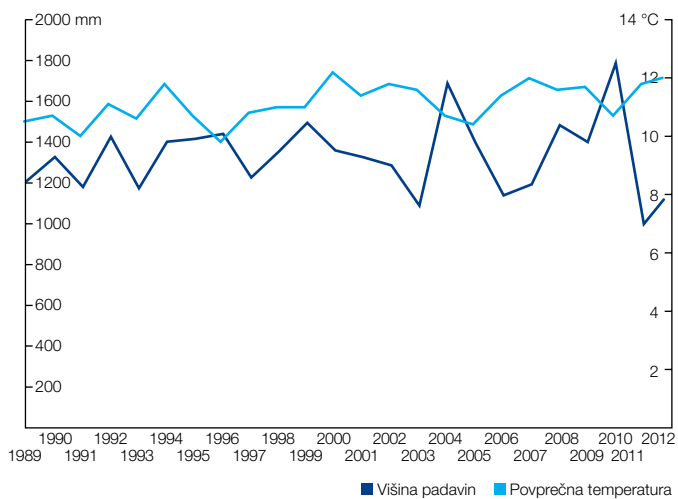
Letna višina padavin in povprečne temperature zraka v letih 1989–2012
