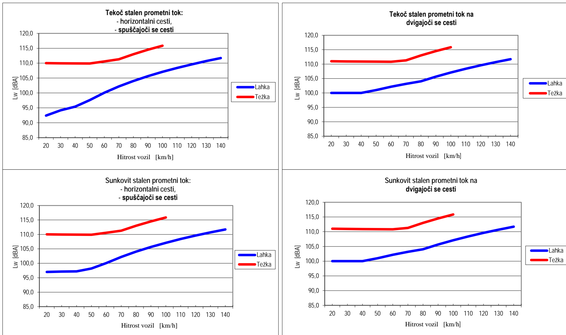
Slika 3: Normirana zvočna moč L_w posameznega vozila glede na hitrost in vzdolžni naklon vozišča za tekoči in za sunkovit stalen promet
