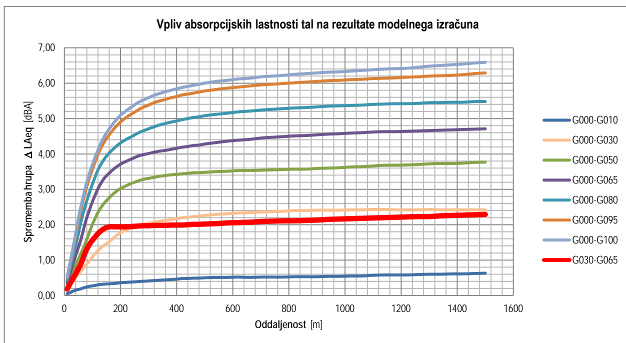
Slika 14: Vpliv absorpcijskih lastnosti tal na širjenje hrupa
