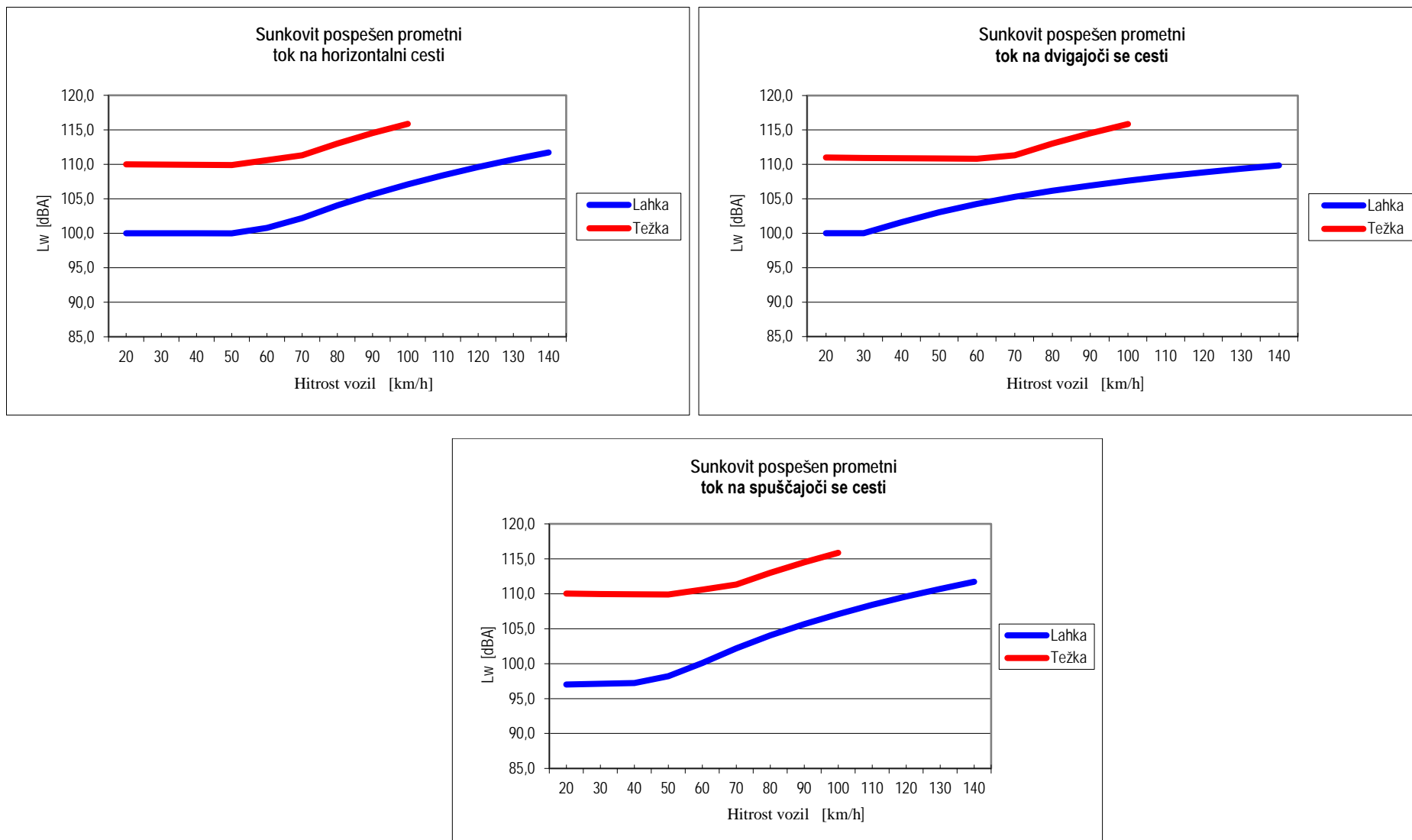
Slika 4: Zvočna moč L_w posameznega vozila glede na hitrost in vzdolžni naklon vozišča za sunkovit pospešen promet
