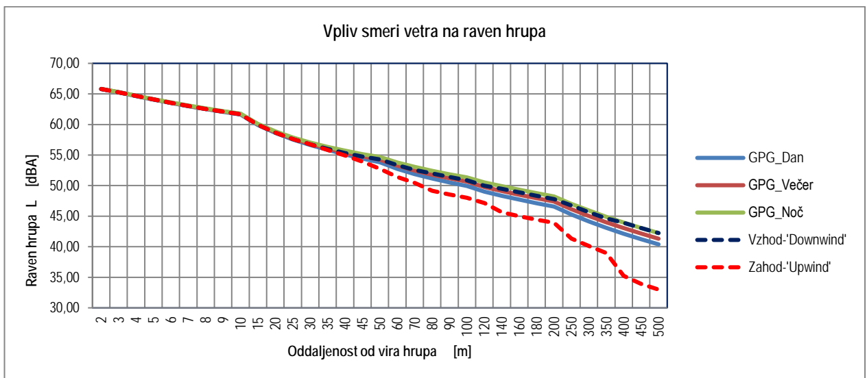
Slika 9: Primerjava rezultatov ocenjevanja po GPG [5] s situacijami "Downwind" in "Upwind"
