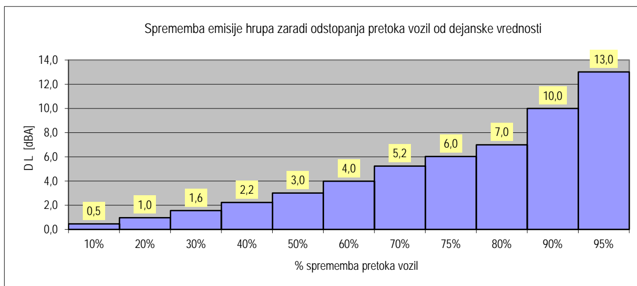
Slika 11: Sprememba emisije ceste kot vira hrupa v odvisnosti od spremembe pretoka vozil
