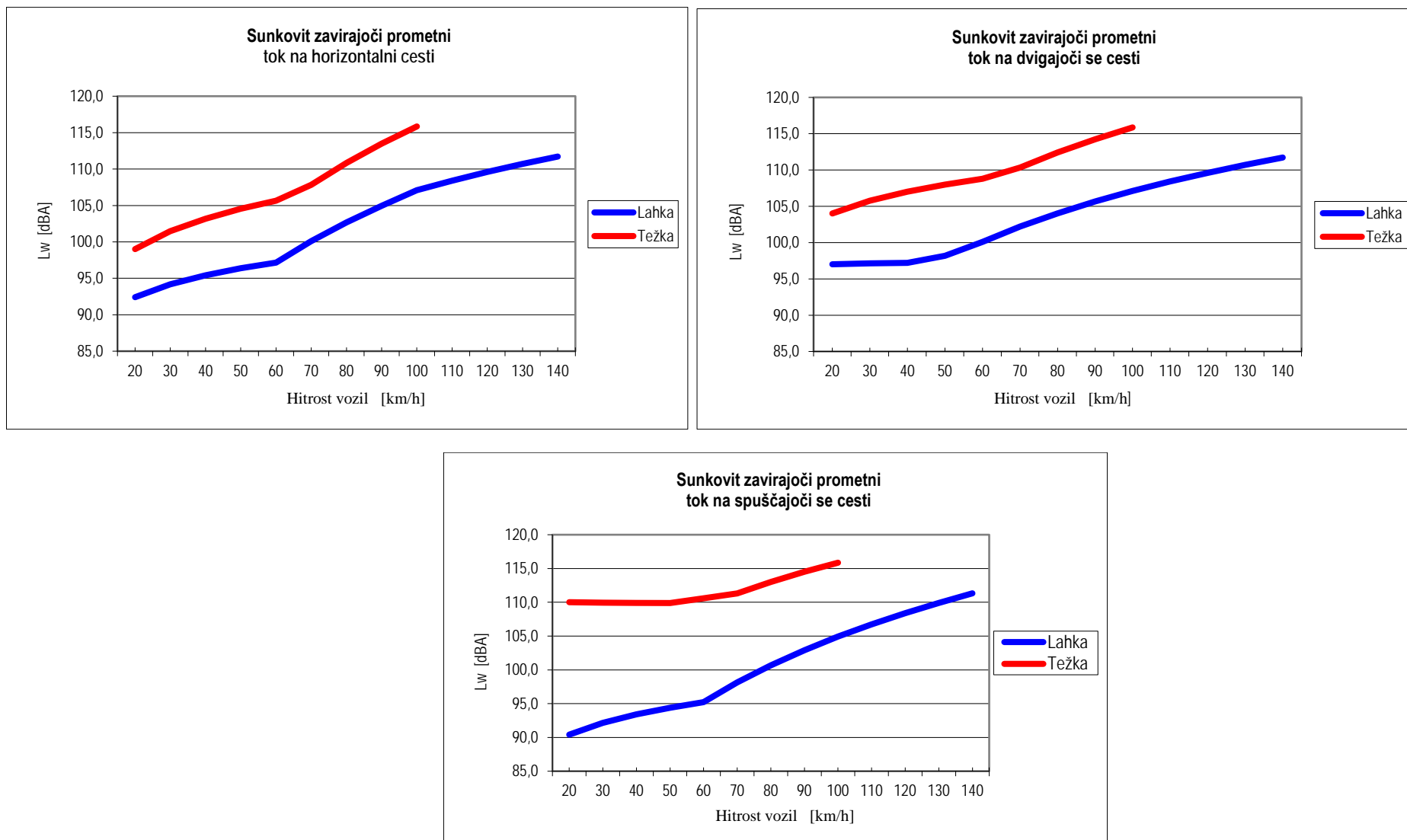
Slika 5: Zvočna moč L_w posameznega vozila glede na hitrost in vzdolžni naklon vozišča, za sunkovit zavirajoči promet
