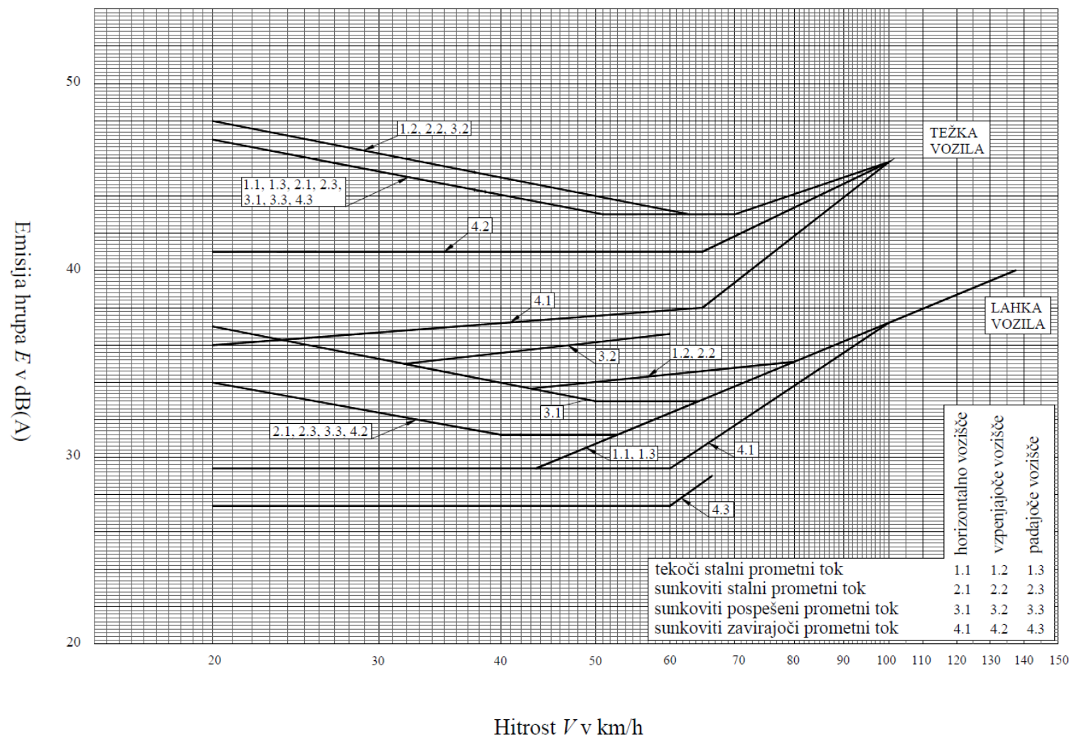
Slika 2: Nomogram za določanje vrednosti emisije hrupa E (vir: Wölfel Meßsysteme Software GmbH)
