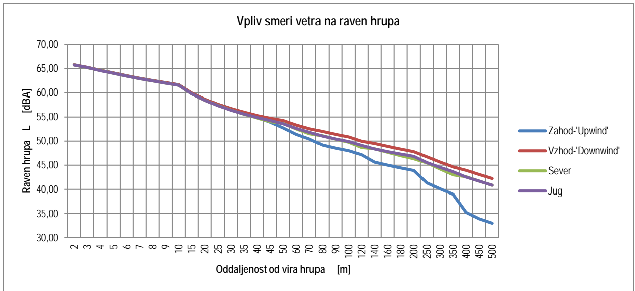
Slika 8: Rezultati računske ocene ravni hrupa glede na za širjenje hrupa ugodnih smeri vetra
