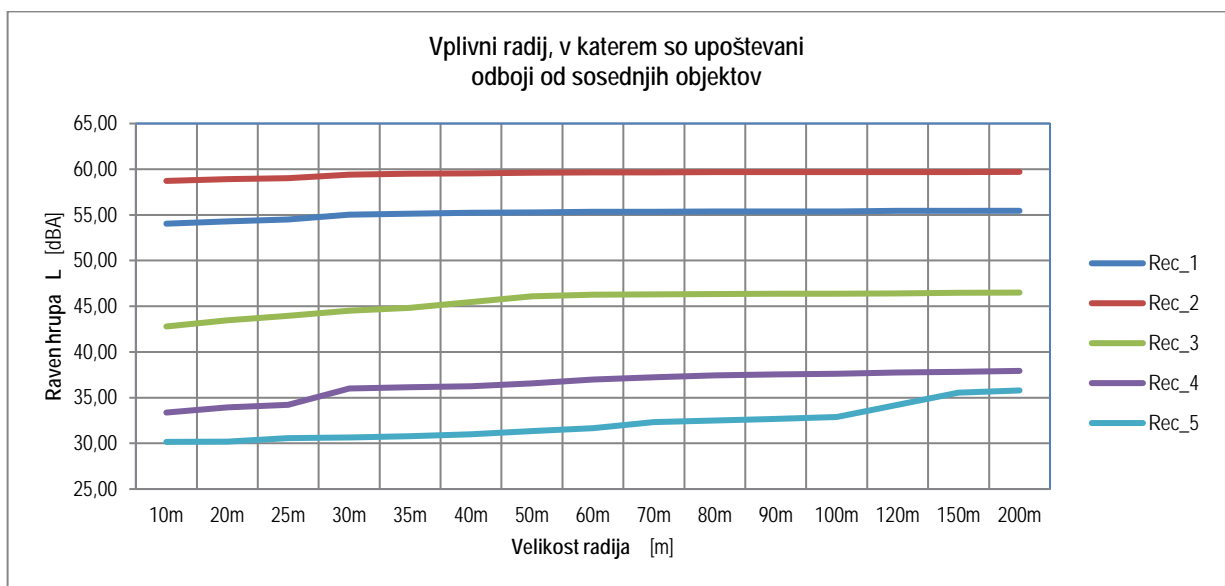
Slika 17: Vpliv velikosti radija, v katerem so upoštevani odboji od sosednjih objektov, na rezultate modelnega izračuna
