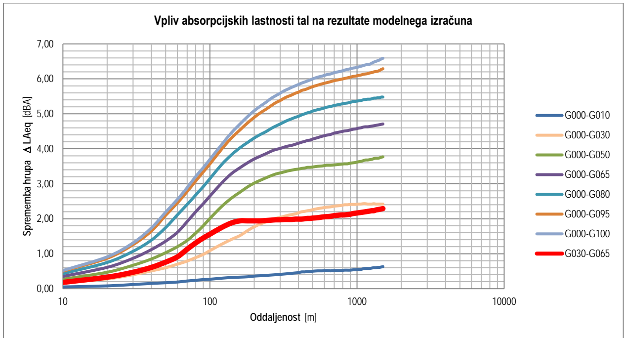
Slika 15: Vpliv absorpcijskih lastnosti tal na širjenje hrupa (op. logaritemsko merilo)
