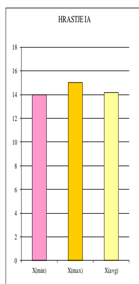
Slika 4: Podzemna voda –Krom VI ( \mu\text{g/l} ), Hrastje IA
