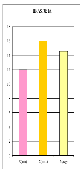
Slika 3: Podzemna voda – Celotni krom ( \mu\text{g/l} ), Hrastje IA
