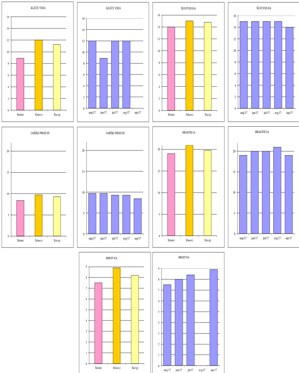
Slika 2: Podzemna voda – Nitrat (mg NO 3 /l)
