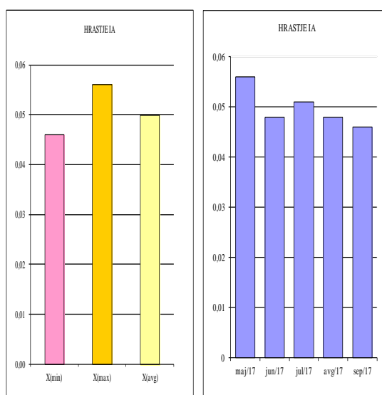
Slika 5: Podzemna voda – Atrazin (µg/l), Hrastje IA
