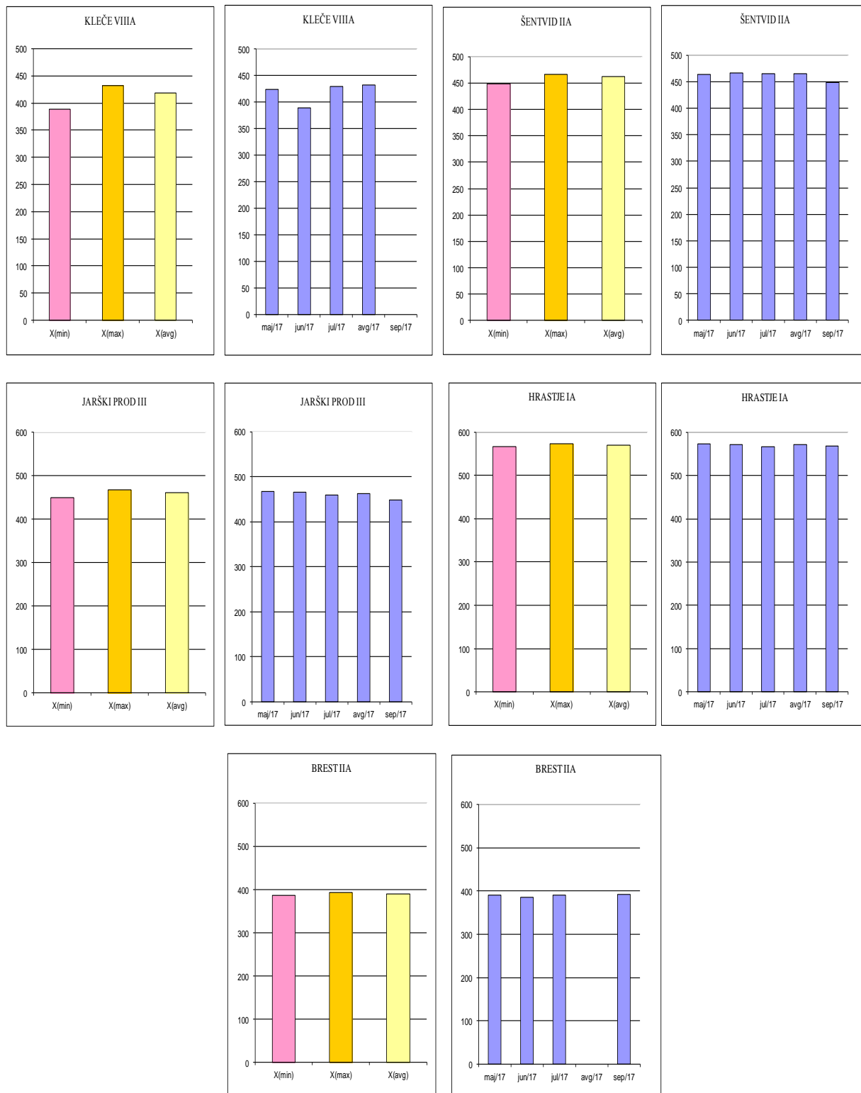
Slika 1: Podzemna voda – Električna prevodnost (pri 20° C, \mu\text{S/cm} )
