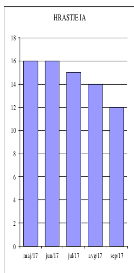
Slika 3: Podzemna voda – Celotni krom ( \mu\text{g/l} ), Hrastje IA
