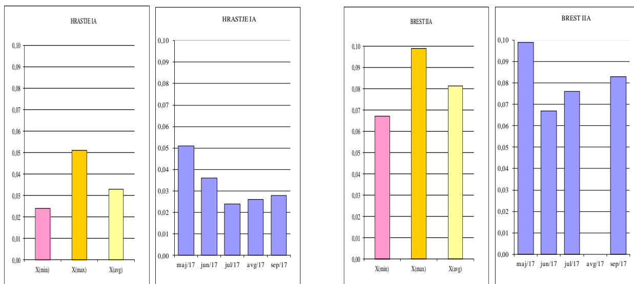
Slika 6: Podzemna voda – Desetilatrazin (µg/l), Hrastje IA Slika 7: Podzemna voda – Desetilatrazin (µg/l), Brest IIA
