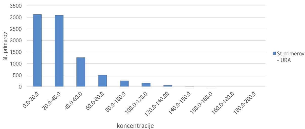
ferkvenčna porazdelitev koncentracij \text{PM}_{10}
