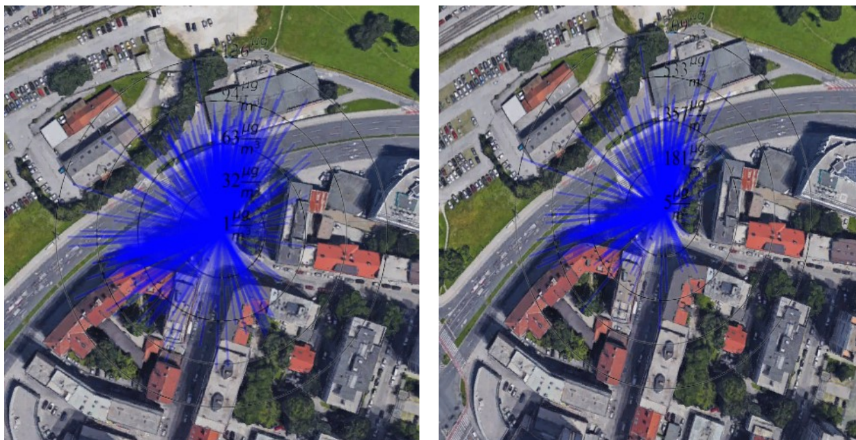
Slika 5: Podrobnejša roža onesnaženja za \text{NO}_2 (levo) in \text{NO}_x (desno) (Vir: Google Earth, 2018)
