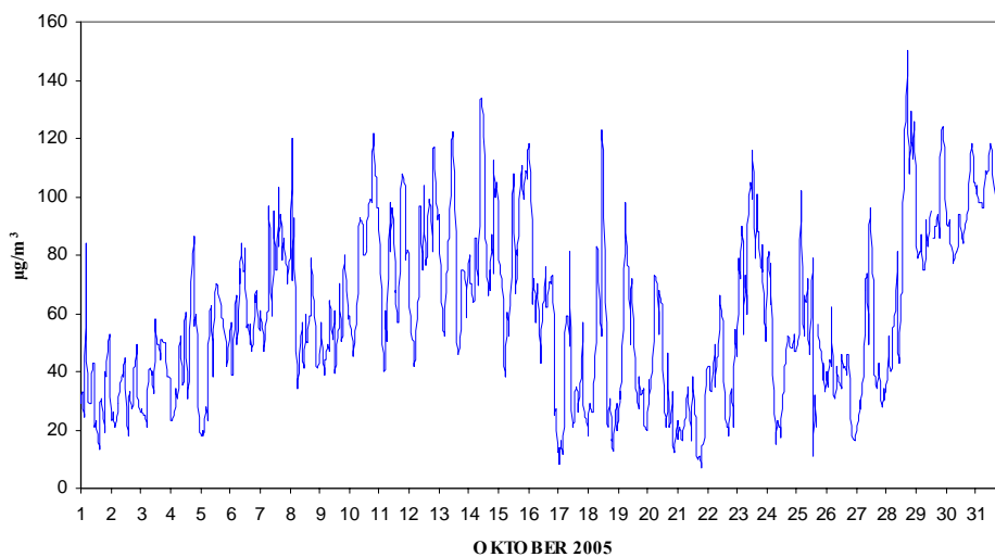
FIGOVEC URNE KONCENTRACIJE DELCEV PM 10
