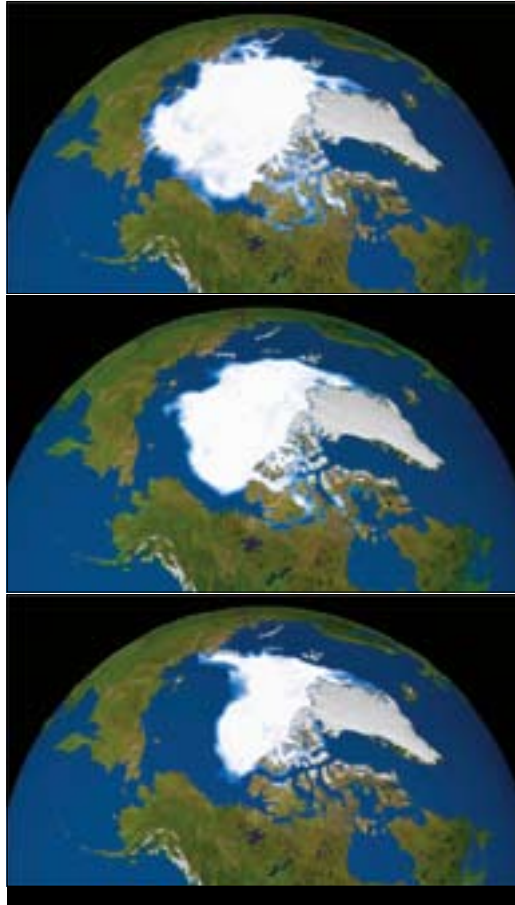
Posnetki pospešenega taljenja arktičnega ledu, hladilnika planeta, v letih 1980, 2005 in 2007.
