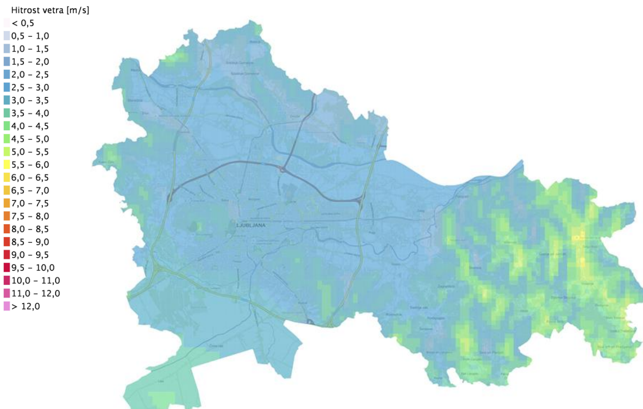
Slika 69: Ocenjena povprečna letna hitrost vetra 50 m nad tlemi na območju MOL na podlagi podatkov Svetovnega vetrnega atlasa (Global Wind Atlas).
