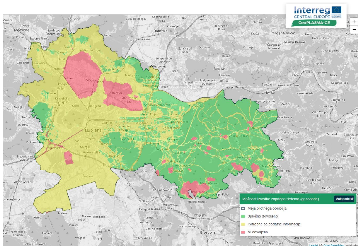
Slika 61: Možnost izvedbe zaprtega sistema na območju MOL.
