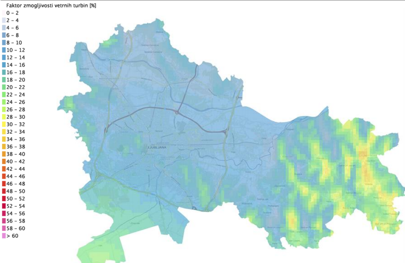
Slika 71: Ocenjen faktor zmogljivosti vetrnih turbin III. razreda po IEC klasifikaciji v MOL na podlagi podatkov Svetovnega vetrnega atlasa (Global Wind Atlas).
