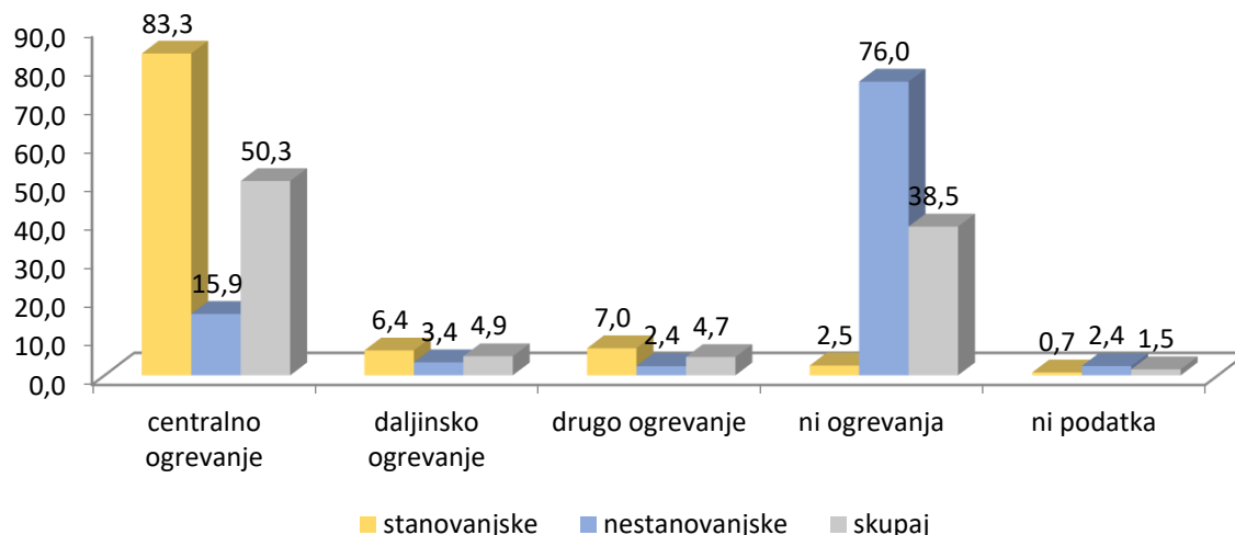
Grafikon 9: Stavbe glede na način ogrevanja v MOL (%).
