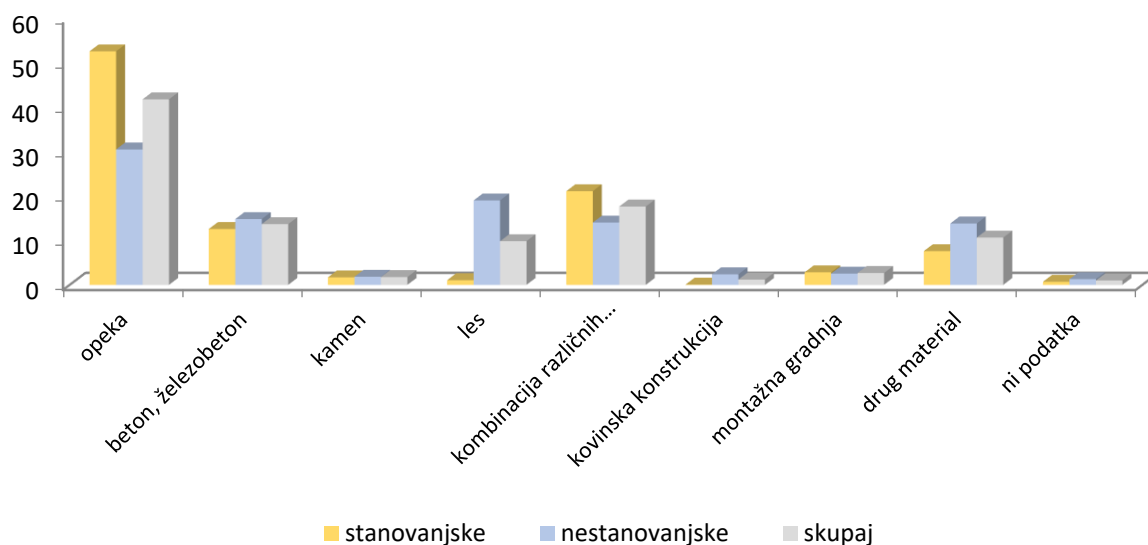
Grafikon 3: Stavbe glede na material nosilne konstrukcije v MOL (%).
