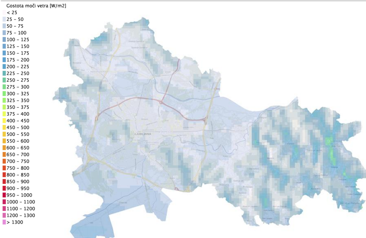
Slika 70: Ocenjena povprečna letna gostota moči vetra 50 m nad tlemi na območju MOL na podlagi podatkov Svetovnega vetrnega atlasa (Global Wind Atlas).
