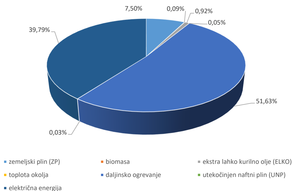
Grafikon 24: Deleži skupne letne rabe energentov za delovanje državnih stavb v Občini Ljubljana.
