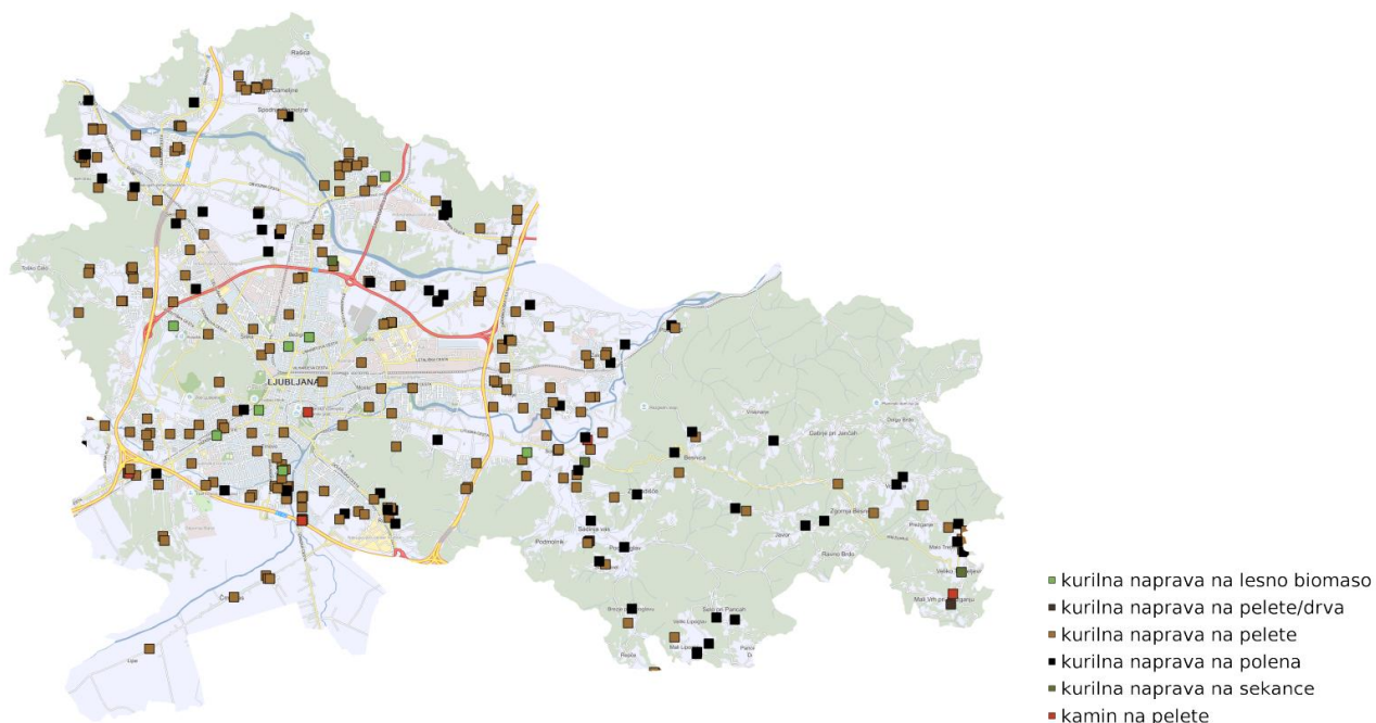
Slika 44: Lokacije kurilnih naprav na lesno biomaso na območju MOL - sofinanciranje s strani Eko sklada, j. s. med letoma 2009 in 2020.
