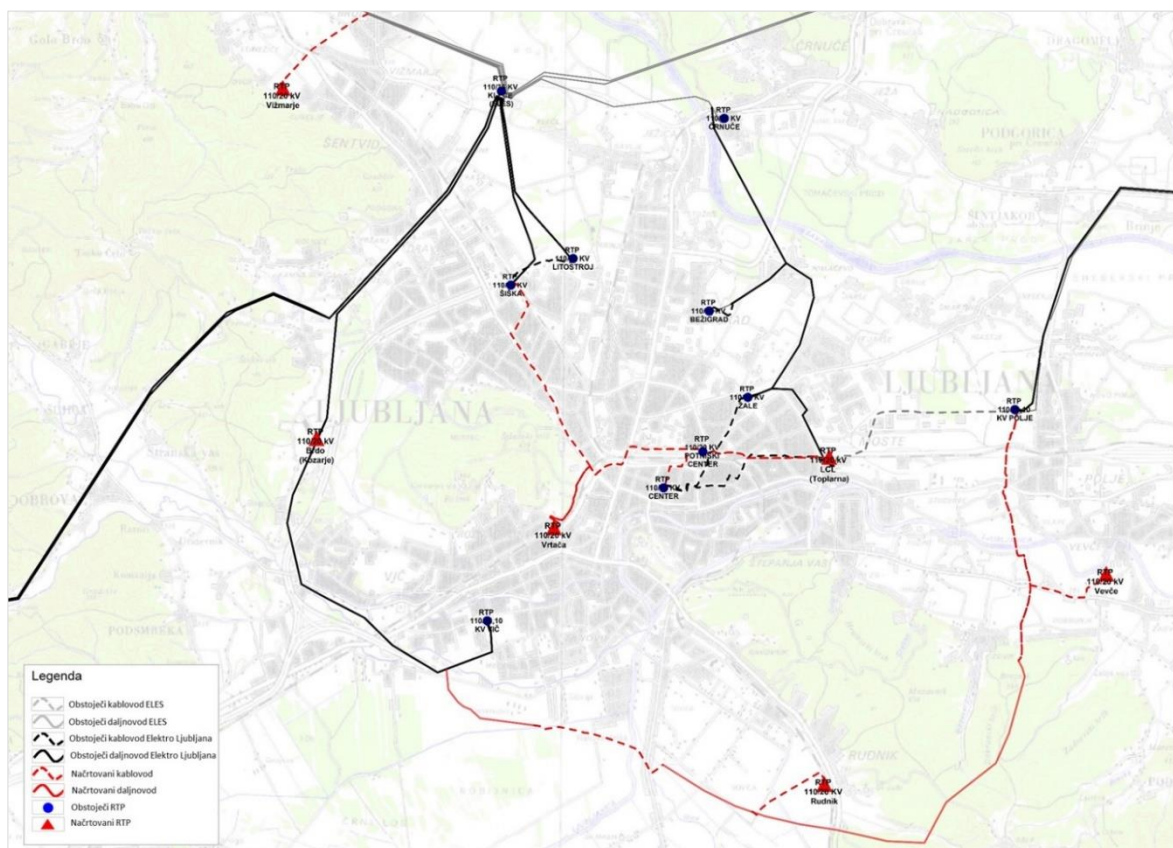
Slika 41: Razvojna geografska shema za 110 kV objekte v MOL.
