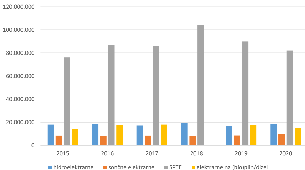
Grafikon 40: Proizvedene količine električne energije po vrsti elektrarn v kWh. Vir podatkov: Elektro Ljubljana, d. d.
