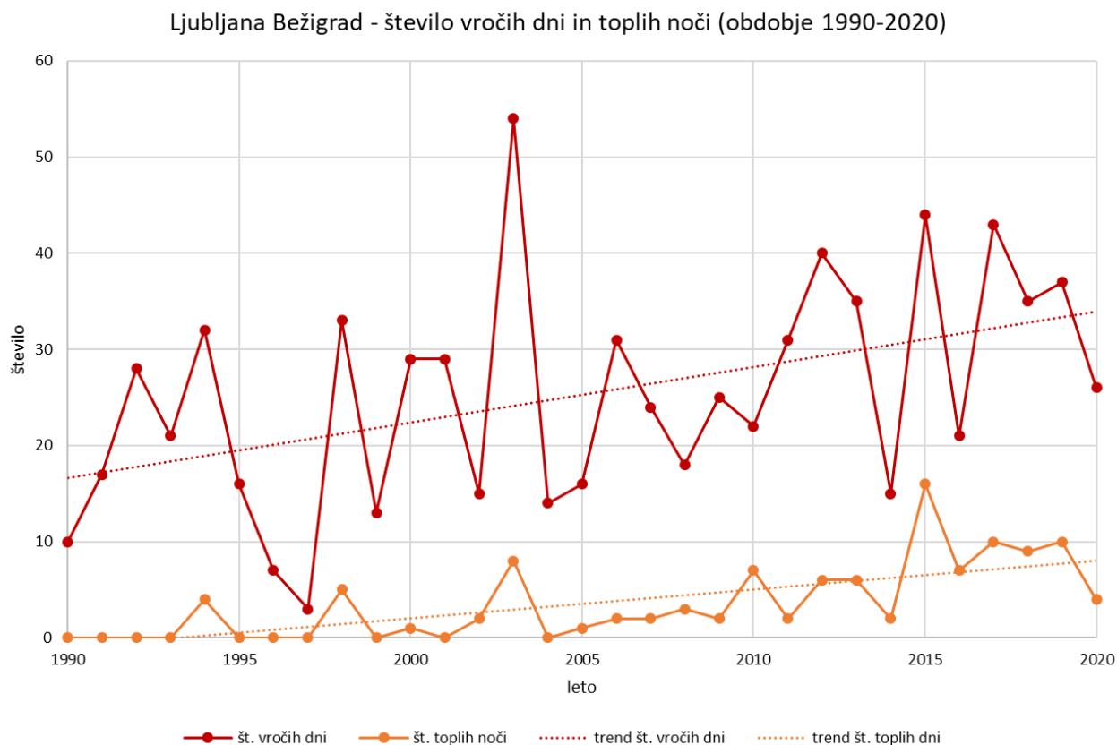
Grafikon 16: Število vročih dni ( T_{maks.} \geq 30\text{ °C} ) in toplih noči ( T_{min.} \geq 20\text{ °C} ) na meteorološki postaji Ljubljana Bežigrad in linearni trend naraščanja.
