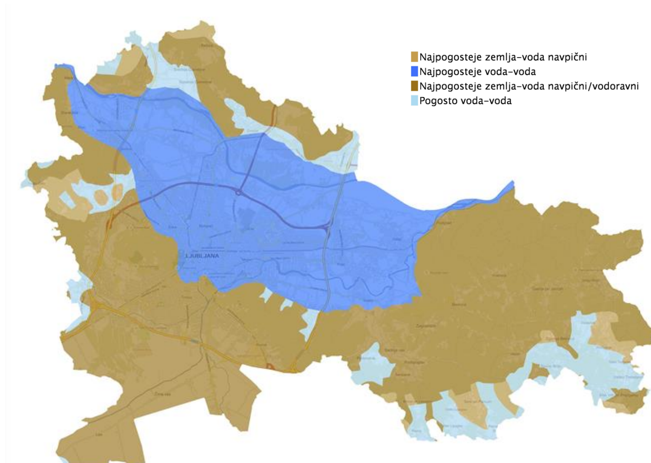
Slika 59: Potencial za geotermalne toplotne črpalke na območju MOL.
