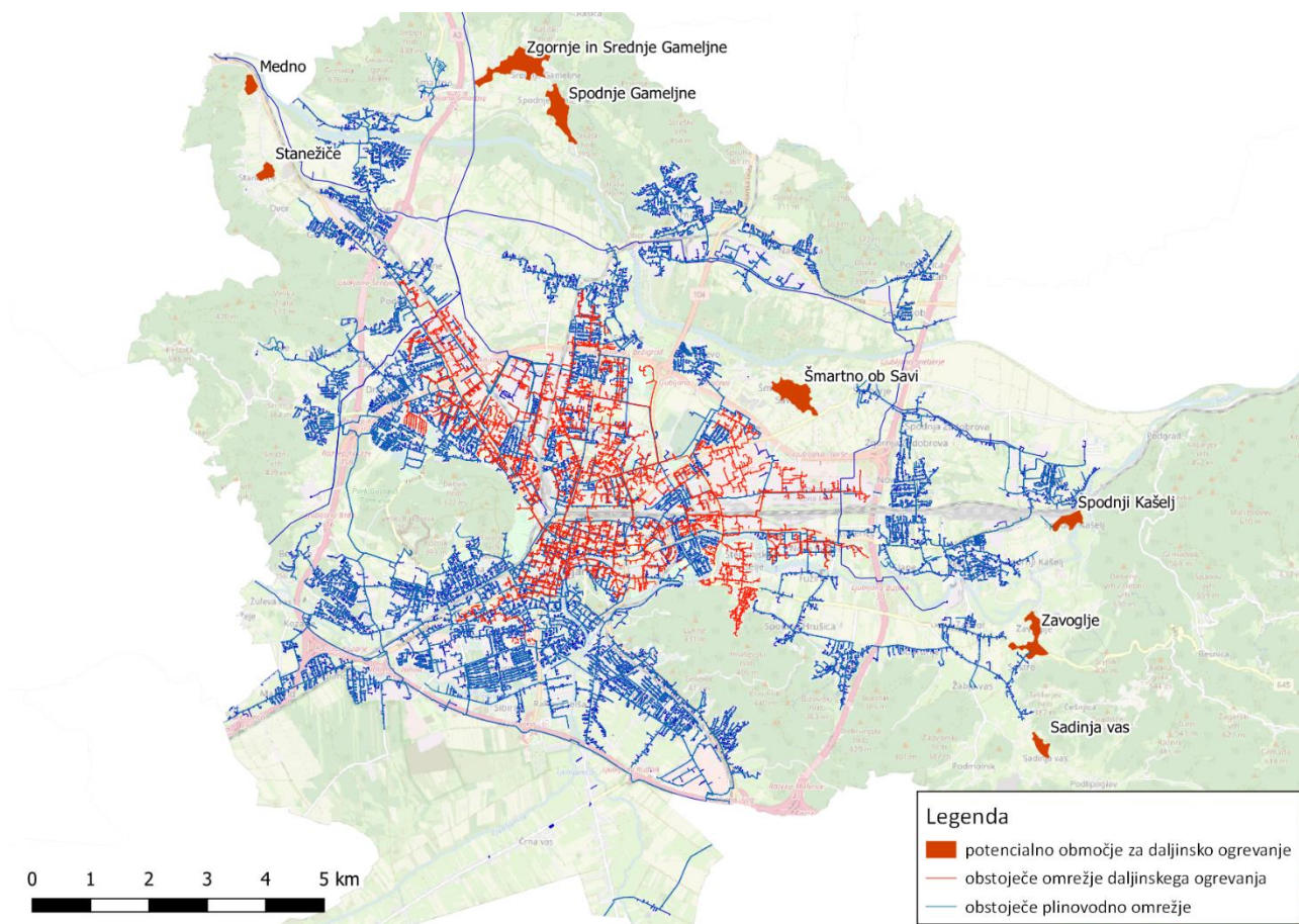
Slika 30: Prikaz potencialnih območij za daljinske sisteme in prikaz obstoječega omrežja daljinskega ogrevanja in zemeljskega plina. Vir: GURS, Envirodual, d. o. o.; kartografska podlaga: OpenStreetMap.
