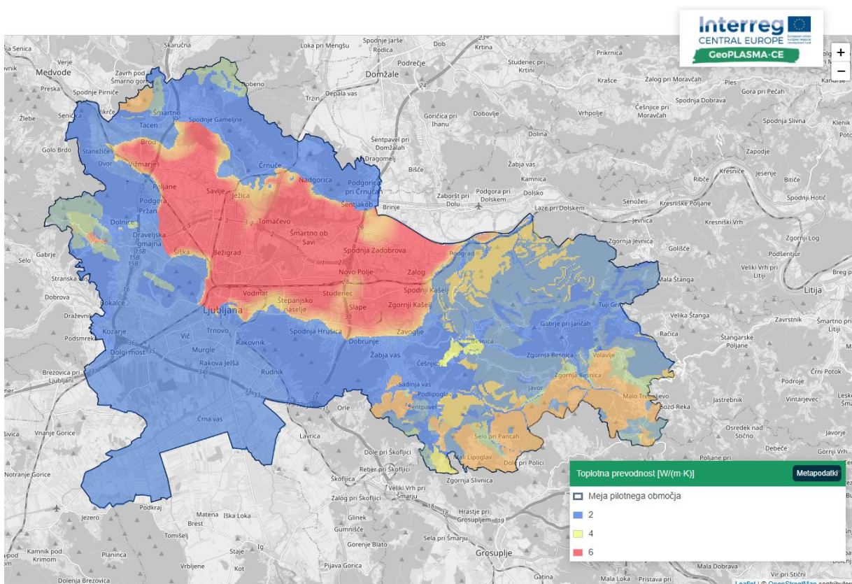
Slika 66: Povprečna celotna toplotna prevodnost od površja do globine 100 m na območju MOL.
