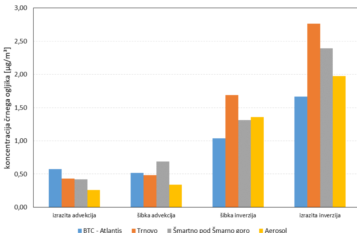
Grafikon 45: Mediana dnevnih koncentracij črnega ogljika iz gorenja biomase na merilnih lokacijah v MOL glede na vremenske tipe v obdobju 2019-2020. Vir podatkov: Aerosol d. o. o.
