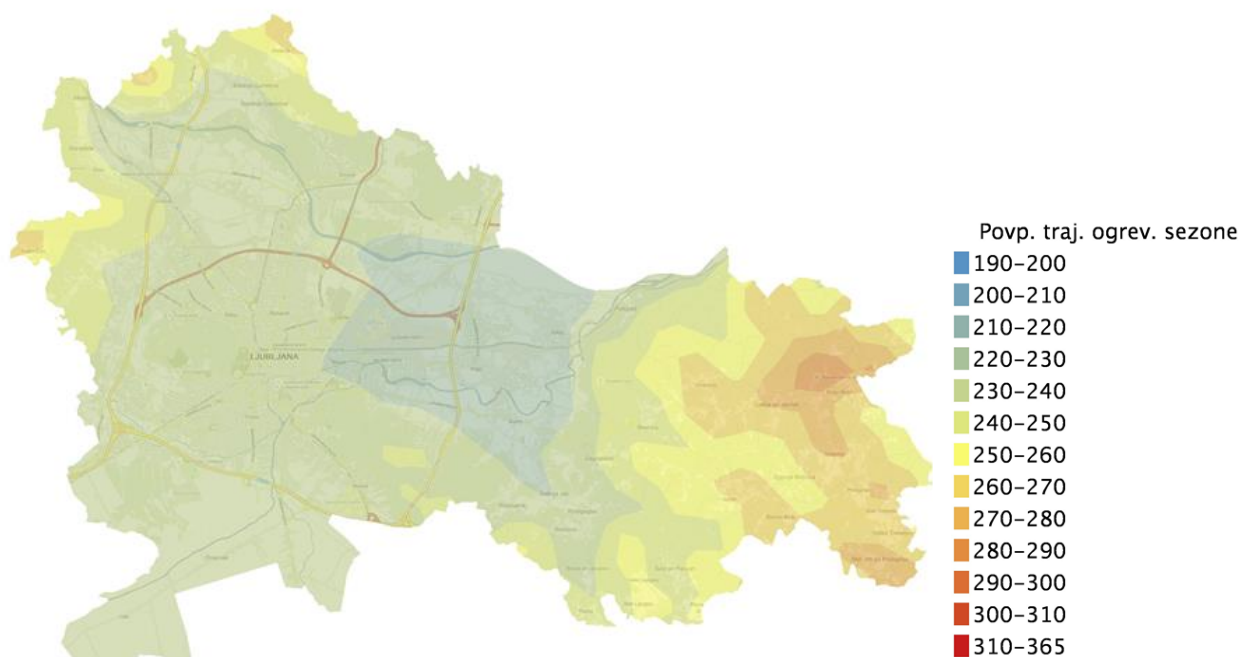
Slika 9: Povprečno trajanje ogrevalne sezone (dni) 1971/72 – 2000/01 v MOL. Vir podatkov: ARSO, kartografija Monolit d. o. o.
