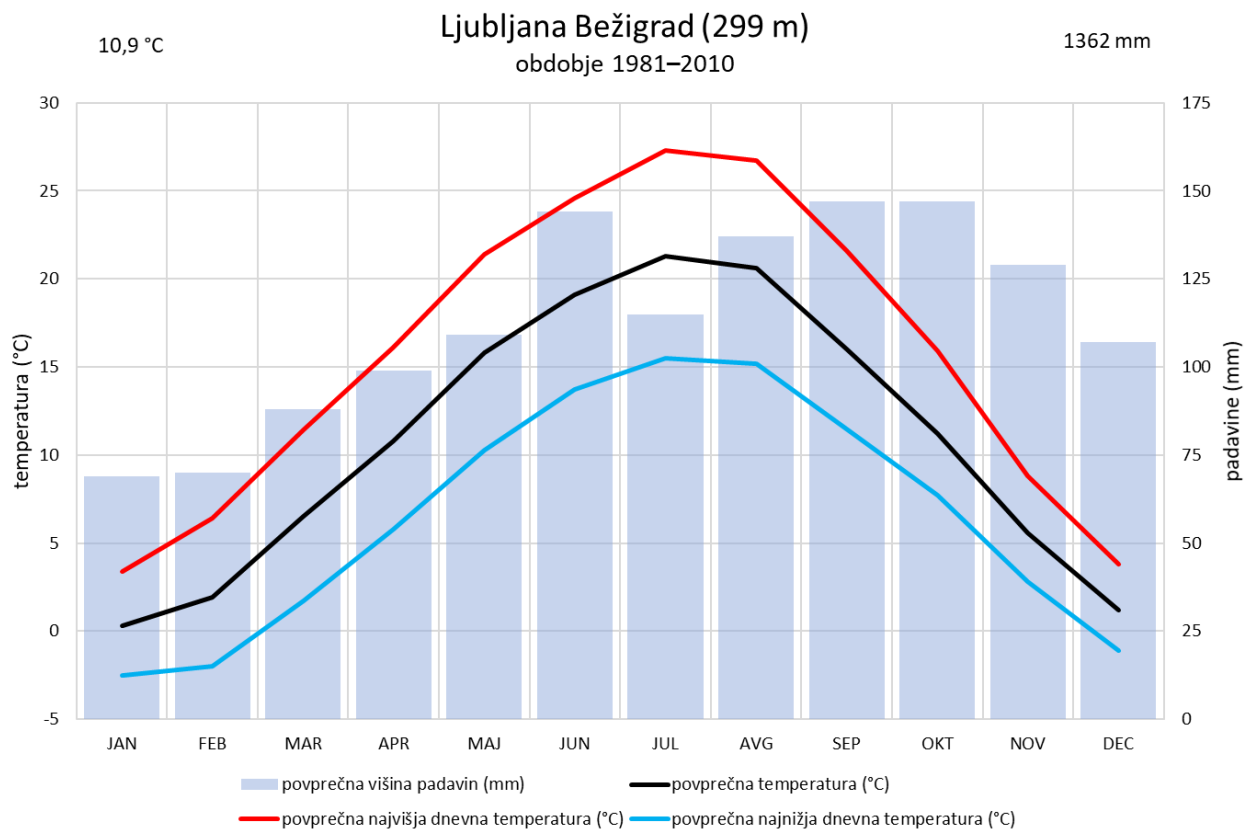
Grafikon 13: Klimogram za meteorološko postajo Ljubljana Bežigrad za referenčno obdobje 1981–2010. Vir podatkov: ARSO.
