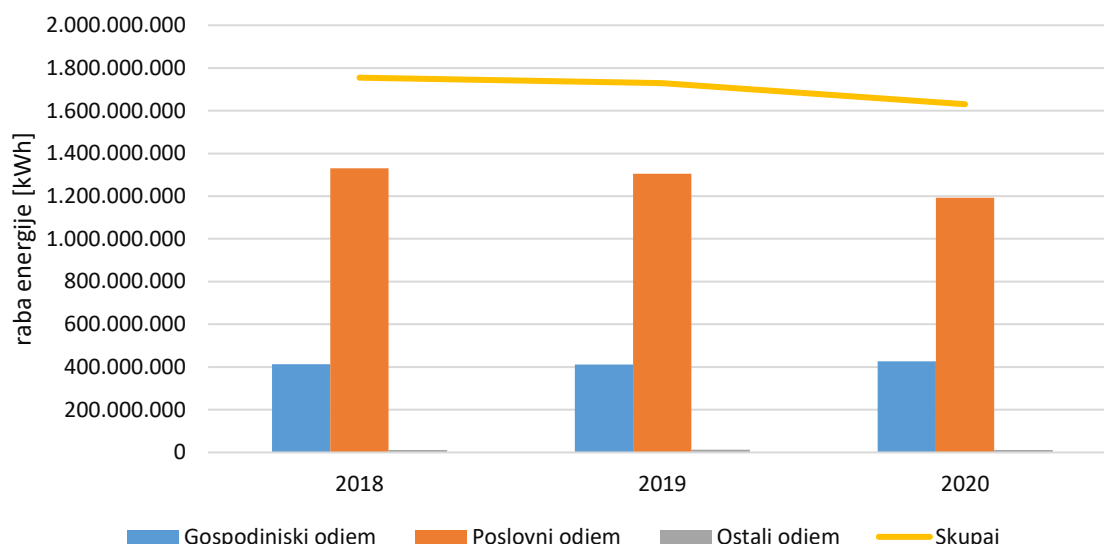
Grafikon 31: Raba električne energije (kWh) v MOL v obdobju 2018–2020 po tarifnih skupinah.
