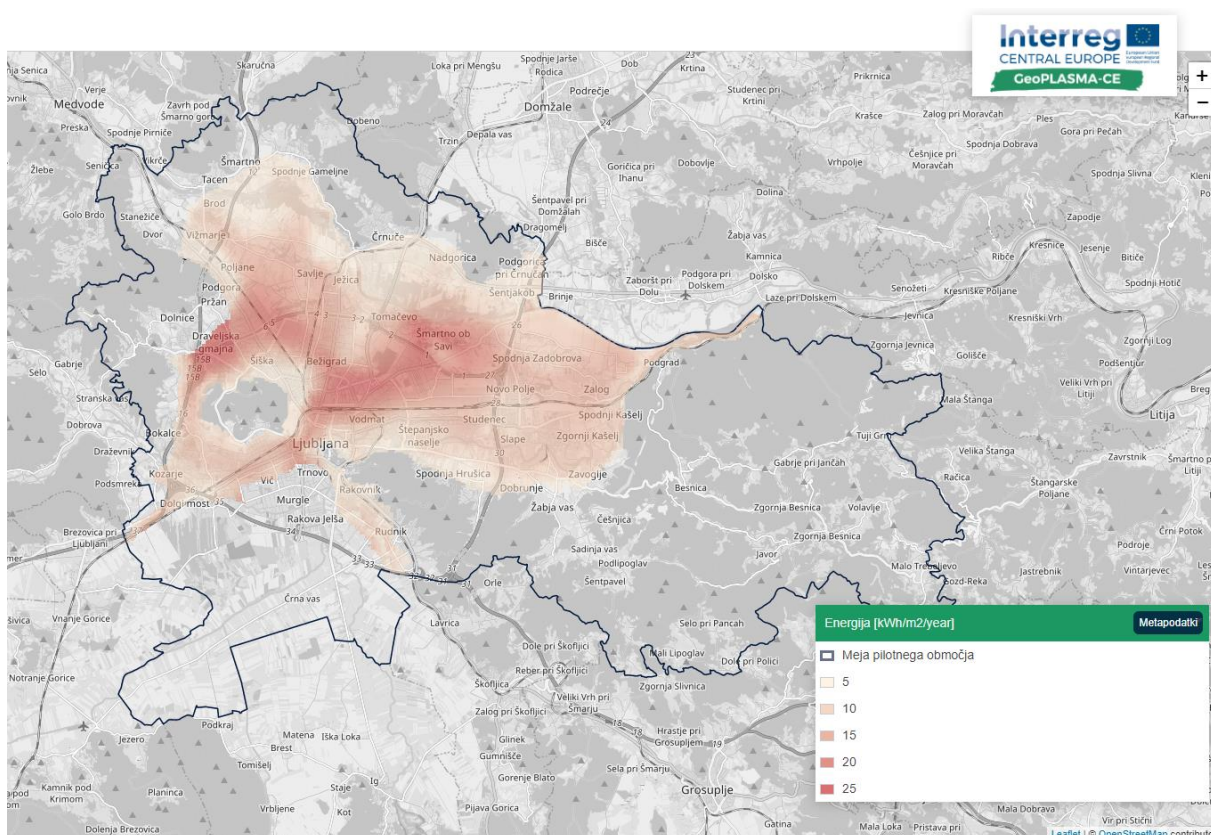
Slika 64: Razpoložljiva energija za ogrevanje z odprtimi sistemi na območju MOL.
