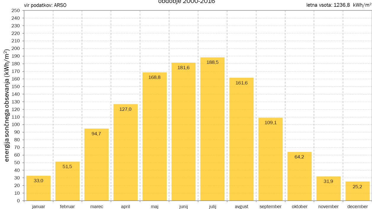
Grafikon 46: Povprečna mesečna energija globalnega sončnega obsevanja na meteorološki postaji Ljubljana Bežigrad v obdobju 2000-2016. Vir podatkov: ARSO.
