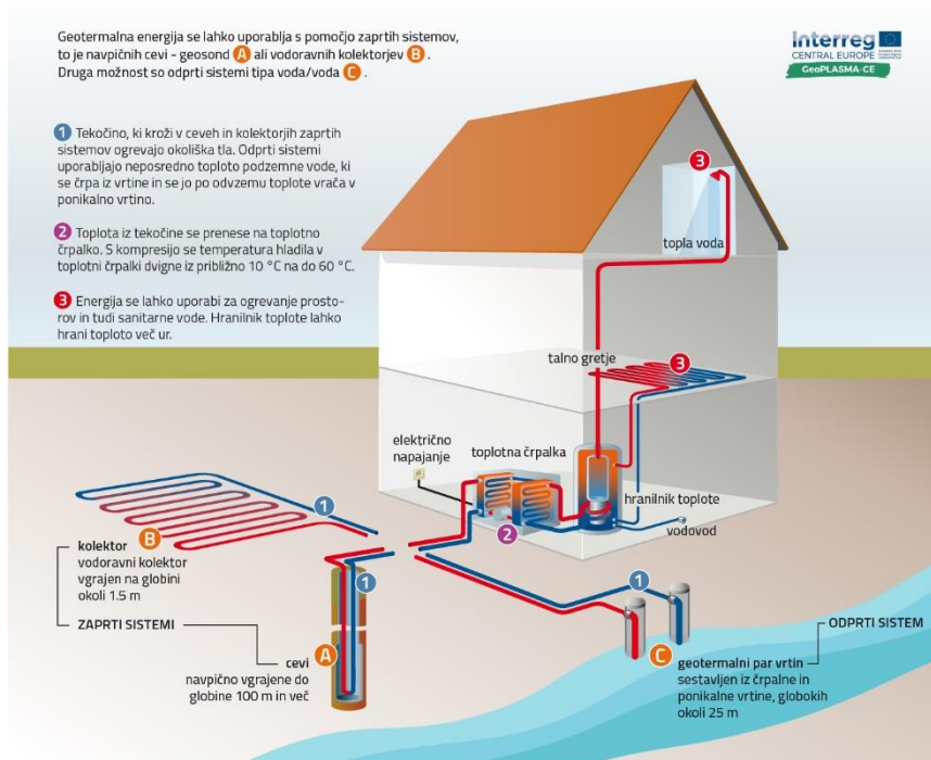
Slika 54: Shematski prikaz delovanja zaprtega in odprtega sistema za izrabo plitve geotermalne energije.
