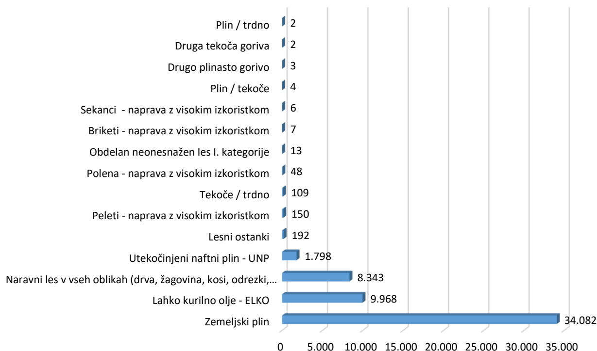
Grafikon 11: Število malih kurilnih naprav glede na energent v MOL.
