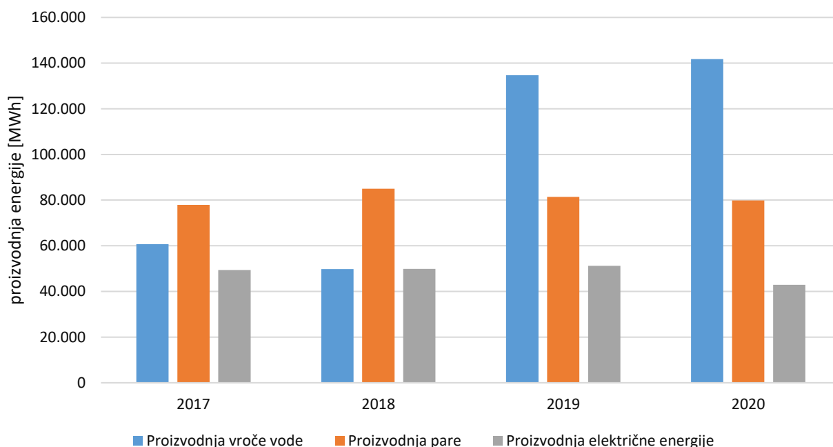
Grafikon 37: Proizvodnja vroče vode, pare in električne energije v TOŠ za obdobje 2017-2020.
