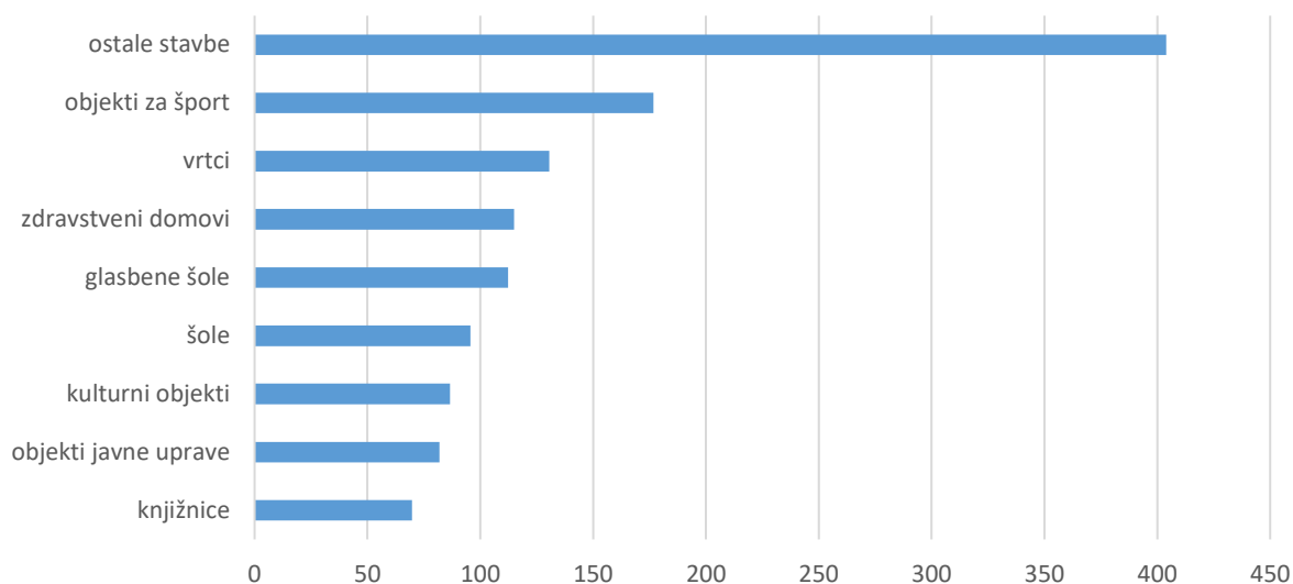
Grafikon 21: Specifična poraba toplote (kWh/m²) javnih stavb v MOL.
