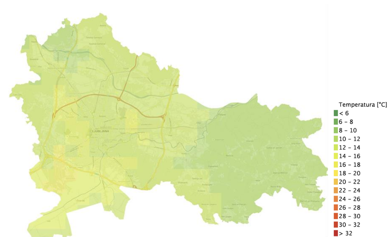
Slika 57: Temperatura v globini 100 m na območju MOL. Vir: GeoZS, kartografija Monolit d. o. o.
