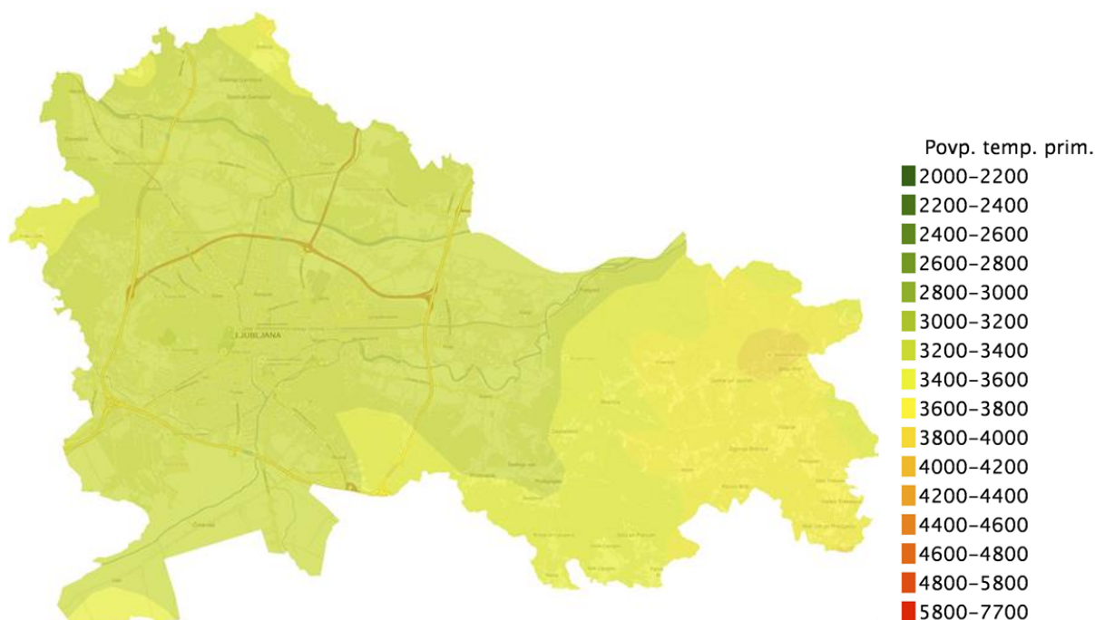
Slika 10: Povprečni temperaturni primanjkljaj (Kdan) 1971-2001 v MOL. Vir podatkov: ARSO, kartografija Monolit d. o. o.
