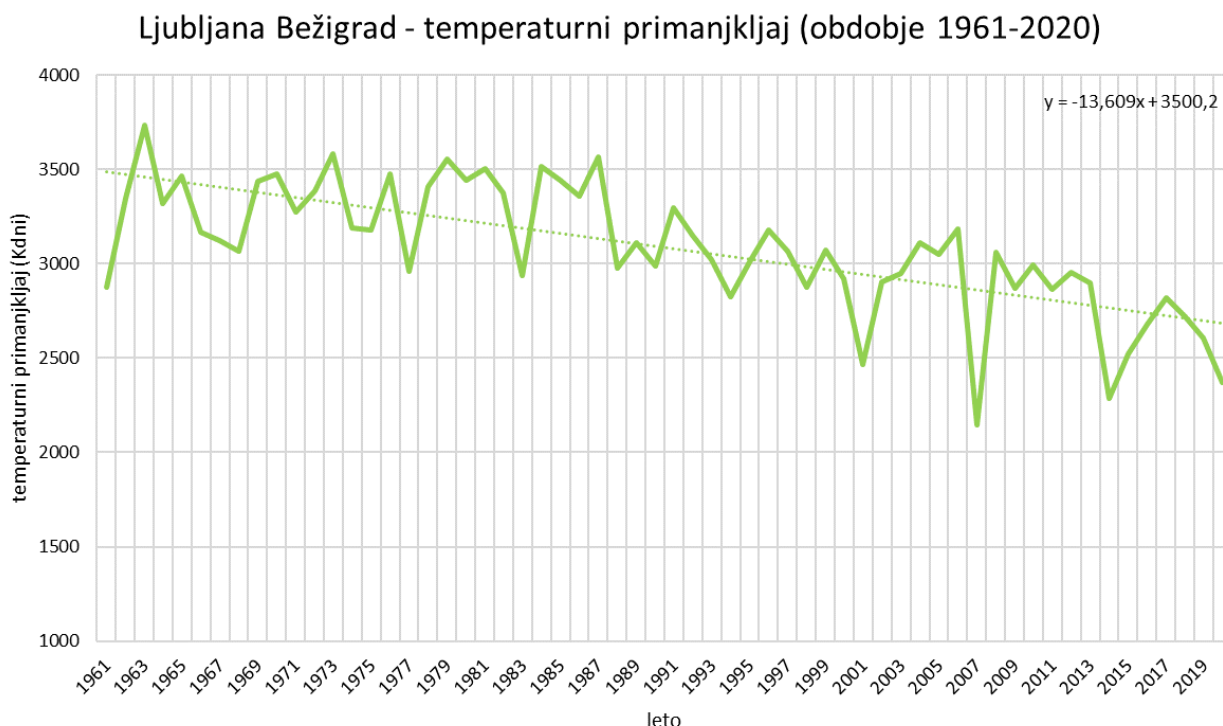
Grafikon 18: Temperaturni primanjkljaj v obdobju 1961-2020 na meteorološki postaji Ljubljana Bežigrad. Vir podatkov: ARSO.
