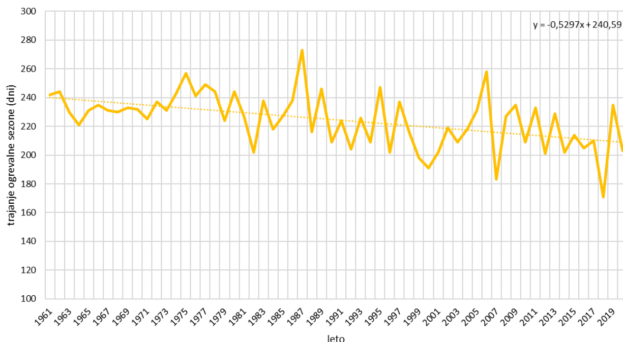
Grafikon 17: Trajanje ogrevalne sezone v obdobju 1961-2020 na meteorološki postaji Ljubljana Bežigrad. Vir podatkov: ARSO.
