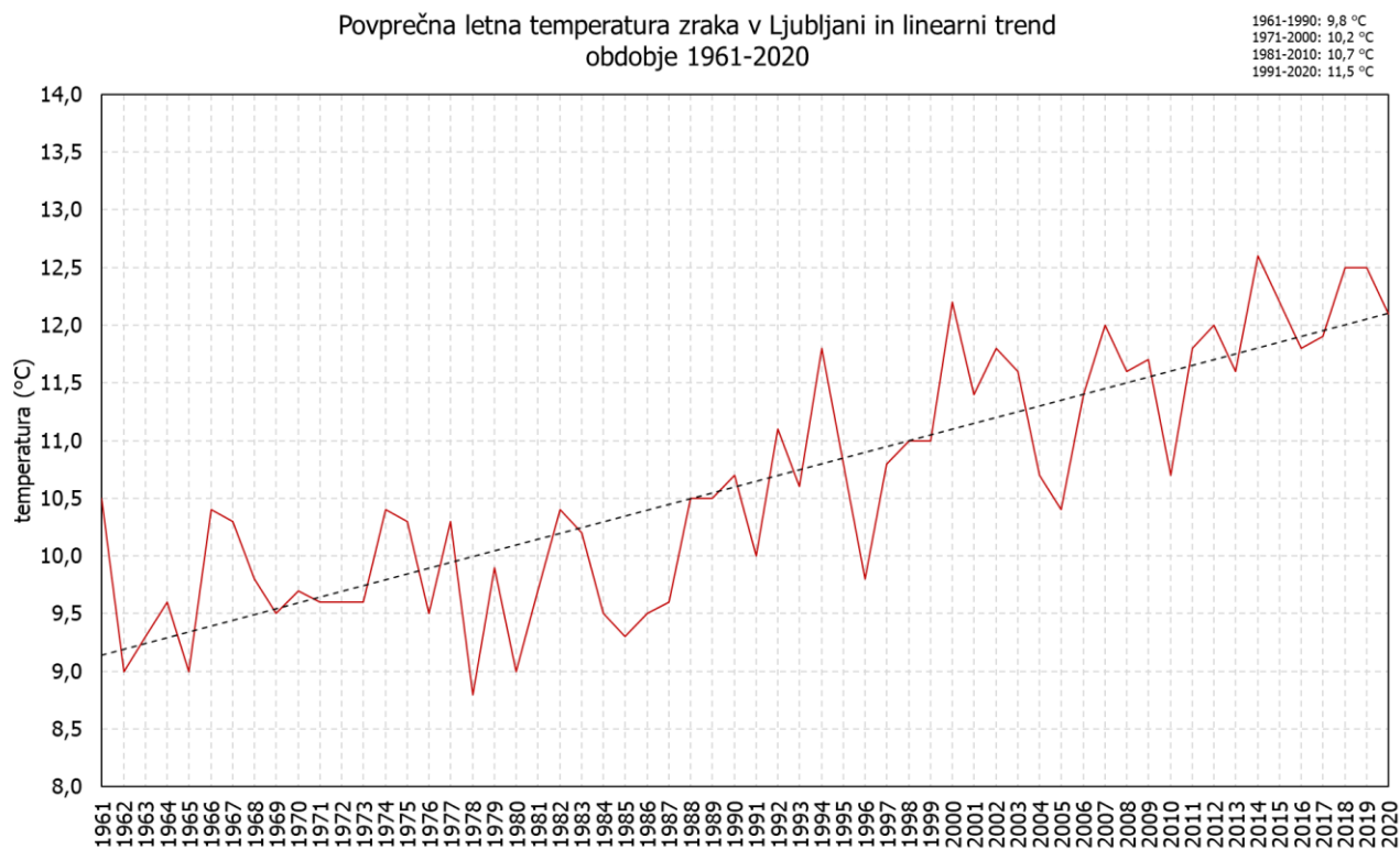
Grafikon 14: Povprečna letna temperatura in linearni trend za meteorološko postajo Ljubljana Bežigrad za obdobje 1961-2020.
