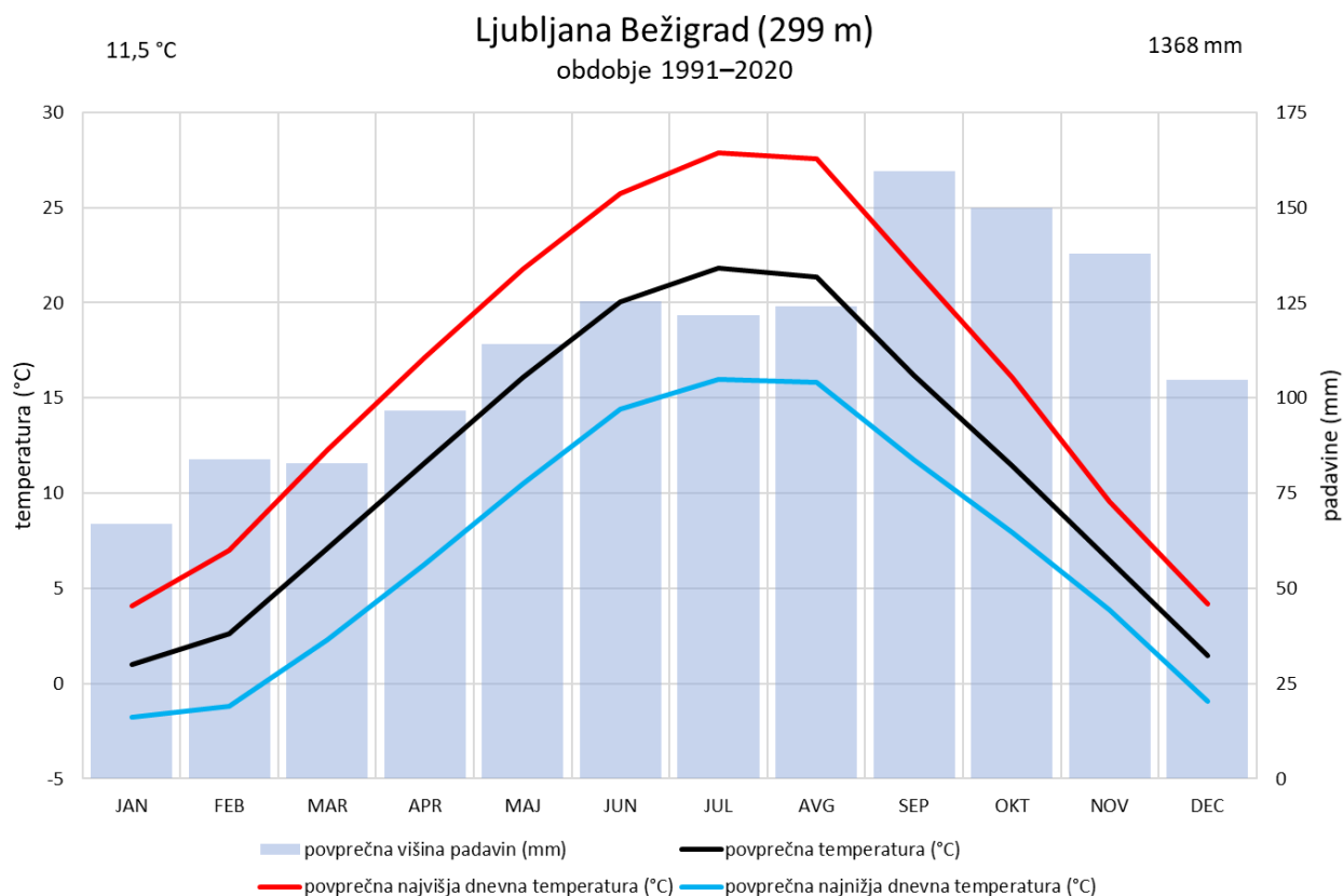
Grafikon 12: Klimogram za meteorološko postajo Ljubljana Bežigrad za obdobje 1991–2020. Vir podatkov: ARSO.
