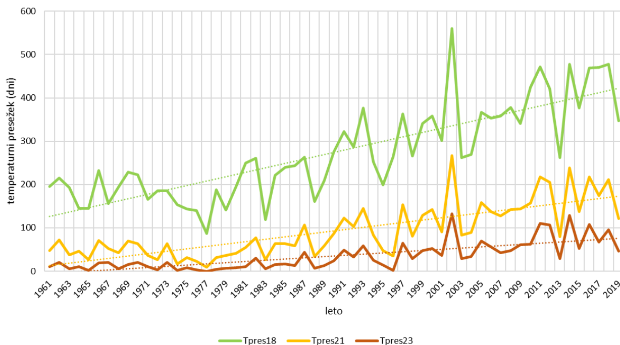
Grafikon 16: Temperaturni presežek za pragove 18, 21 in 23 °C v obdobju 1961-2020 na meteorološki postaji Ljubljana Bežigrad.
