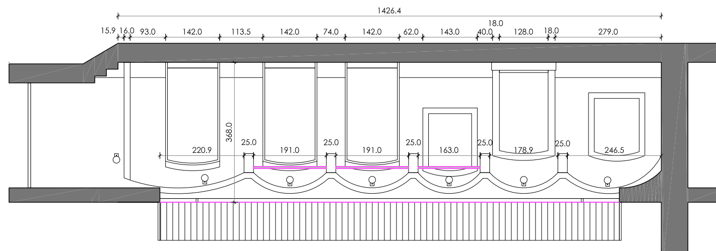
RAZSTAVNI PROSTORI MESTNE HIŠE - DESNI ATRIJ M 1:100
