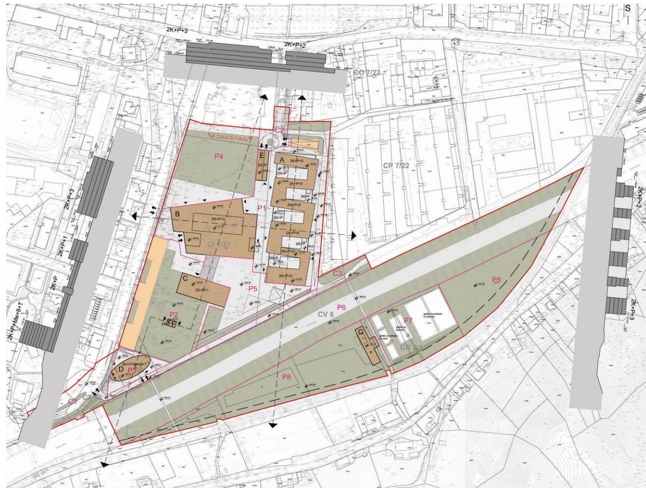
UREDITVENA SITUACIJA STREH IN ZNAČILNI PREREZI SKOZI OBMOČJE
