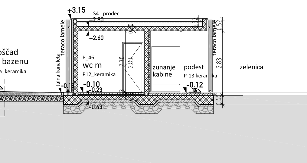
delni prerez e-e
