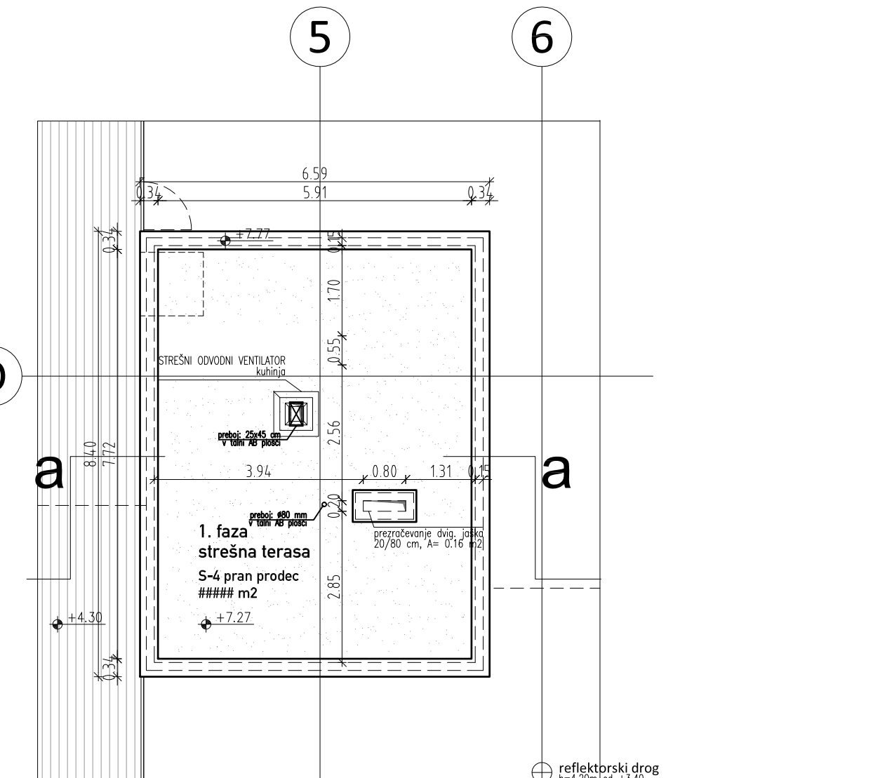
tloris strehe nad stopniščnim jedrom 1:100
