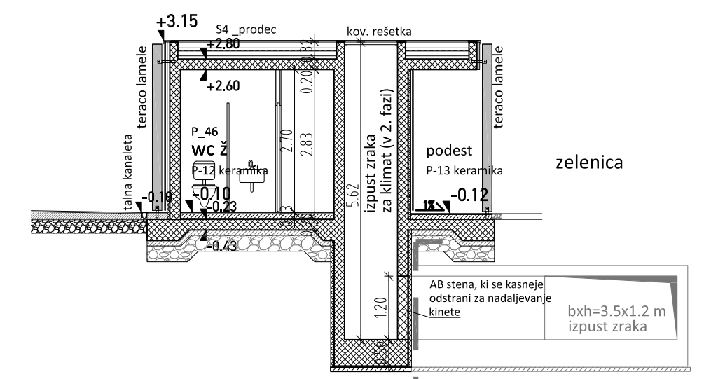
delni prerez e1-e1
