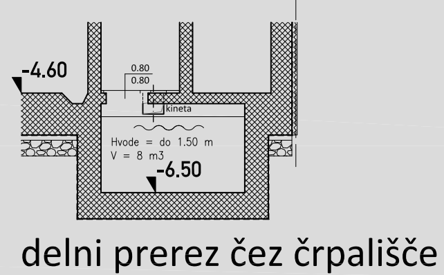
delni prerez čez črpališče
