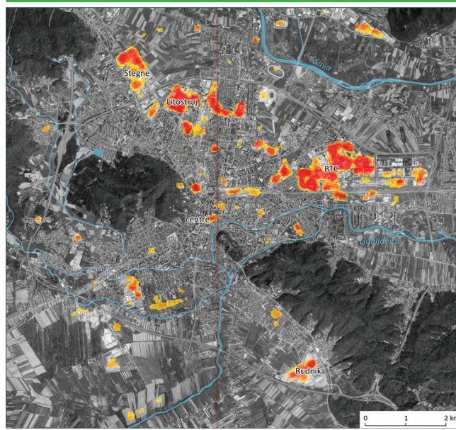
Satelitska termografija
