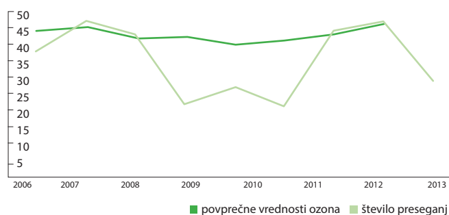
Število preseganj dnevni mejni vrednosti za ozon (Ljubljana Bežigrad, \mu g/m^3 )
