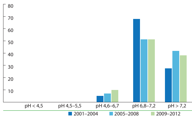
Kislost tal (%)
