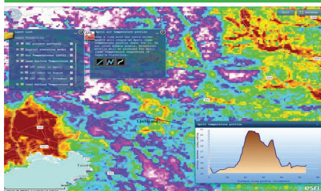
Satelitska termografija
