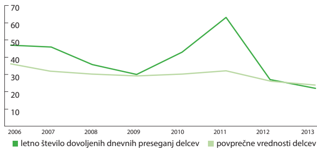
Povprečne vrednosti delcev PM_{10} in letno število dovoljenih dnevni preseganj delcev (Ljubljana Bežigrad, \mu g/m^3 )
