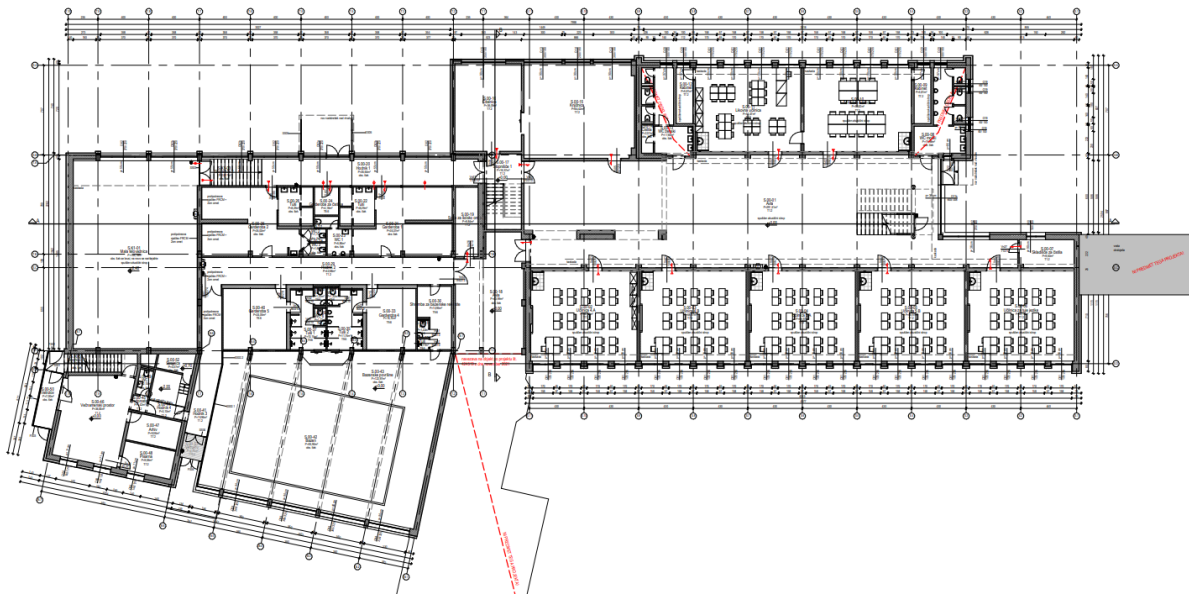
Tloris 2. nadstropja – vzhodni del
