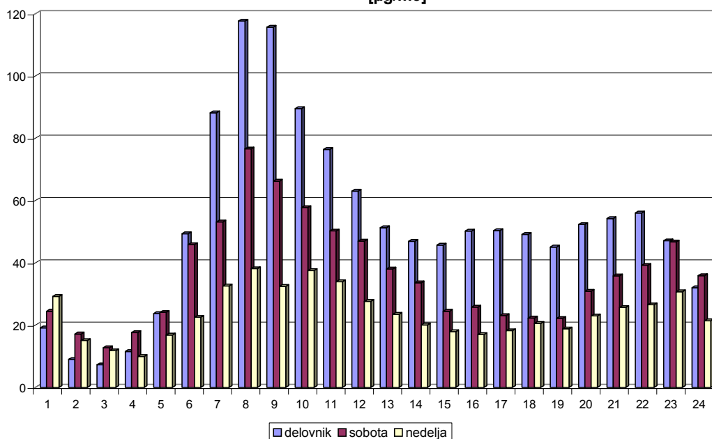
Povprečne koncentracije NO po delovnikih, sobotah in nedeljah izven kurilne sezone v odvisnosti od ure dneva [ \mu\text{g}/\text{m}^3 ]
