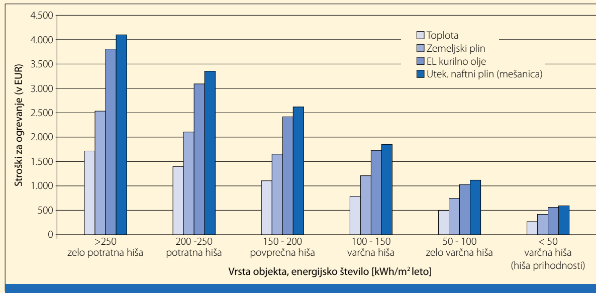
Primerjava letnih stroškov za ogrevanje in pripravo tople vode glede na vrsto objekta oziroma energijsko število.
