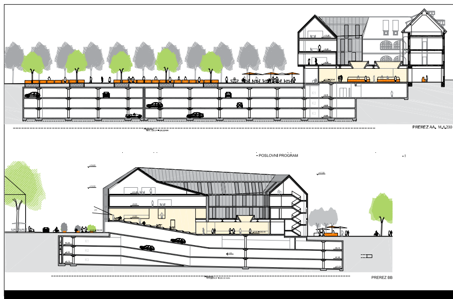
Garažna hiša pod Vodnikovim trgom v prerezu.
