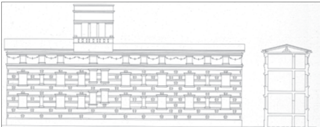
PENSIÓN KOLLMANN M 1/100 Skica dr. FASADE
