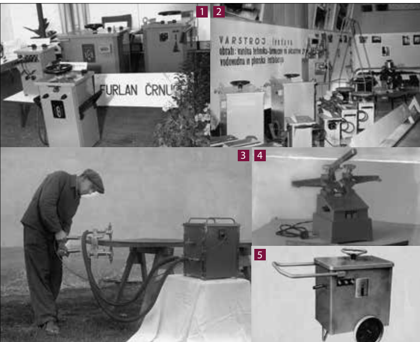
1 Furlanovi izdelki na mednarodni razstavi v Ljubljani 2 Furlanovi izdelki z razstave Varstroj iz Lendave. 3 Točkovno uporovno varjenje. 4 Varilni nadaparator za varjenje tračnih žag. 5 Varilni aparat za obločno varjenje tip 250 A.
