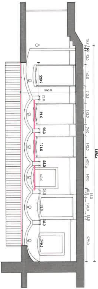
RAZSTAVNI PROSTORI MESTNE HIŠE - DESNI ATRIJ M 1:100
