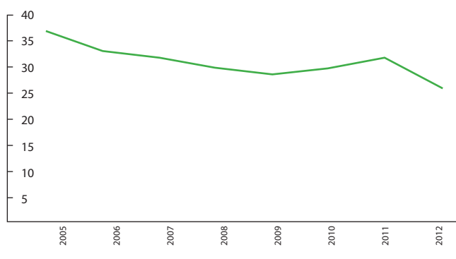
Število preseganj dnevnih mejnih vrednosti za ozon (Ljubljana Bežigrad, \mu g/m^3 )
