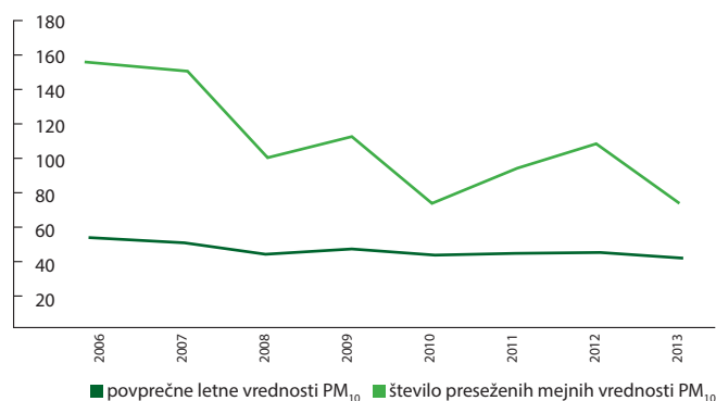
Povprečne vrednosti PM_{10} in letno število dovoljenih dnevnih preseganj delcev (Ljubljana Bežigrad, \mu g/m^3 )
