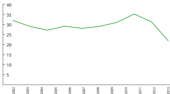
Povprečne vrednosti dušikovega dioksida (Ljubljana Bežigrad, \mu\text{g}/\text{m}^3 )
