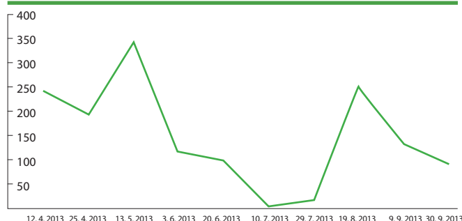
Dinamika nitratnega dušika v tleh rastlinjaka v času rasti plodovk na VVO MOL (kg NO 3 -N/ha)
