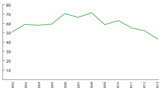
Povprečne vrednosti dušikovega dioksida (Ljubljana Center, \mu\text{g}/\text{m}^3 )
