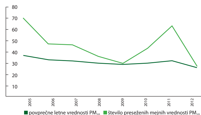
Povprečne vrednosti PM_{10} in letno število dovoljenih dnevnih preseganj delcev (Ljubljana Bežigrad, \mu g/m^3 )
